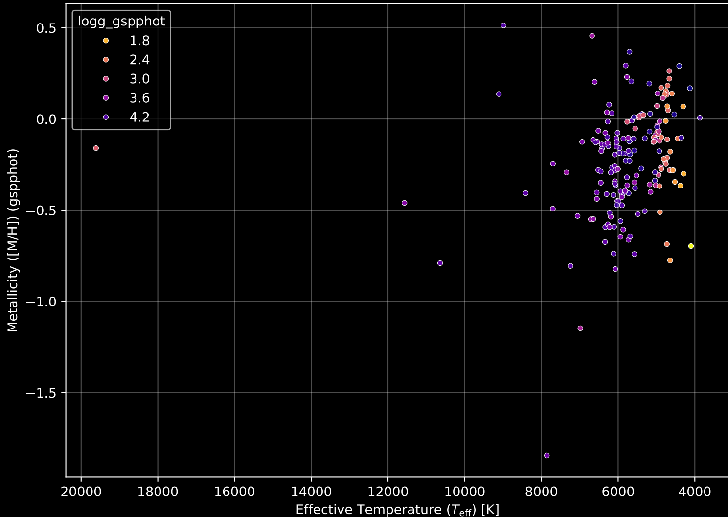
APOGEE DR17 Field: [CVZ_OB10_btx] Stellar Population Parameters (n= 181)
